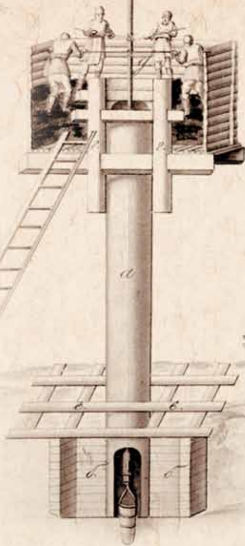
Фрагмент чертежа первоначального устройства рассолоподъемной трубы и загонки матичного дерева. Рисунок из альбома «О каменной соли в Усольских Владельческих солеваренных промыслах открытой», 1831 год.
